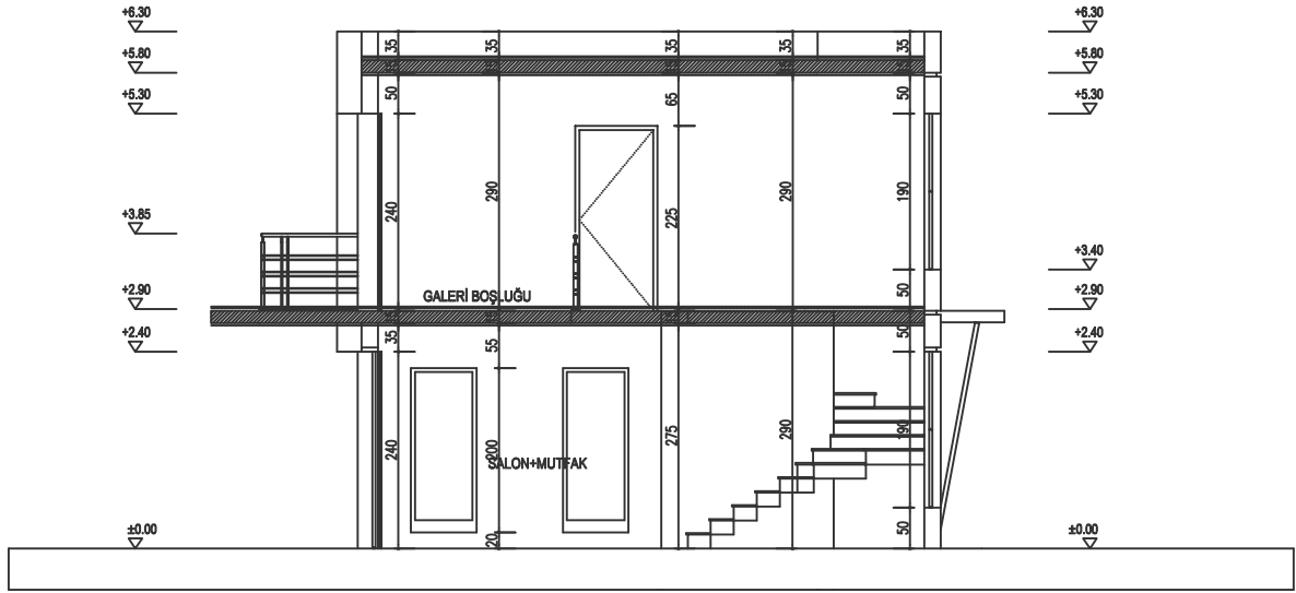
B-B KESİTİ 1/50
