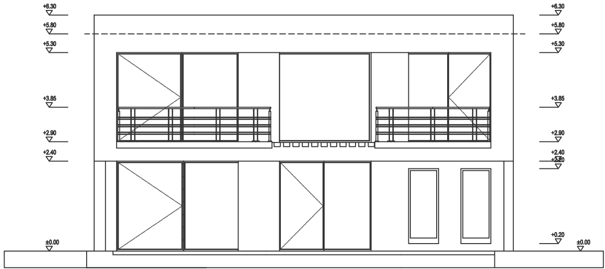
ÖN GÖRÜNÜŞ 1/50
