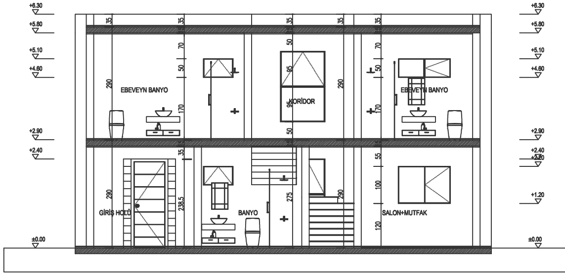
A-A KESİTİ 1/50
