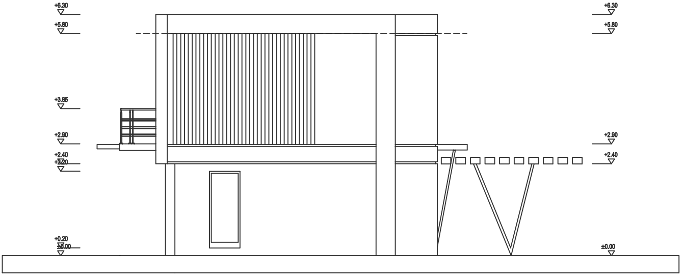
SAĞ YAN GÖRÜNÜŞ 1/50
